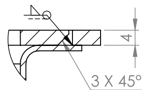
SZCZEGÓŁ B SKALA 1 : 1
