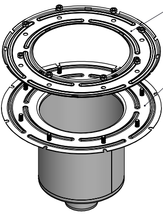
Kołnierz dociskowy Clamping flange
