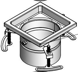
Część górna Upper part
