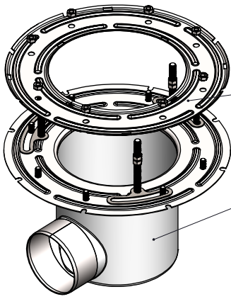
Kołnierz dociskowy Clamping flange
