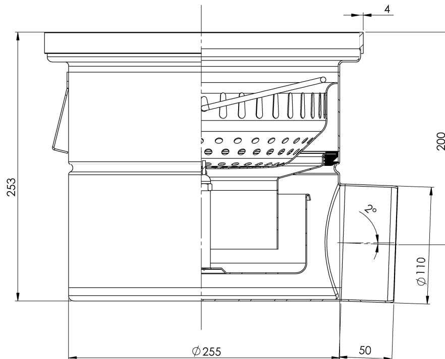
□ Płyta szczelna Tight cover H=25/8mm M125
