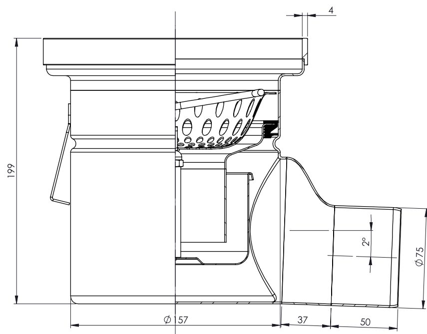
Płyta szczelna Tight cover H=25/8mm M125
