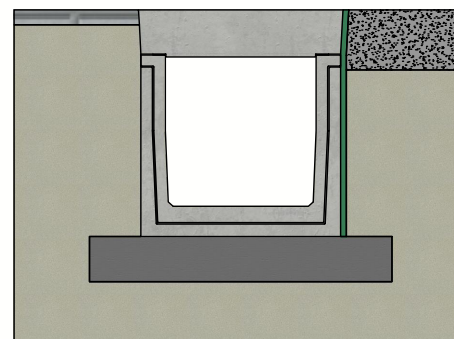
Principe type I (Raadpleeg de plaatsingsvoorschriften)
